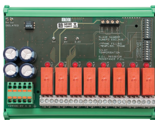
Messwertgeber CPS 10
