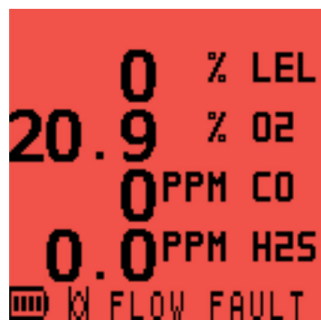
Рисунок 5-8: FLOW FAULT (сбой при отборе пробы)
