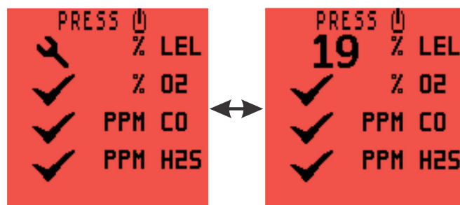
Рисунок 5-3: Сбой LEL ZERO
