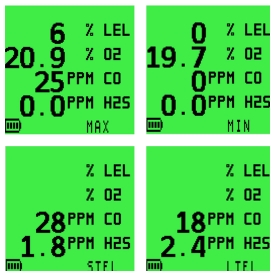
Рисунок 3-14: Значения MAX / MIN / STEL / LTEL
