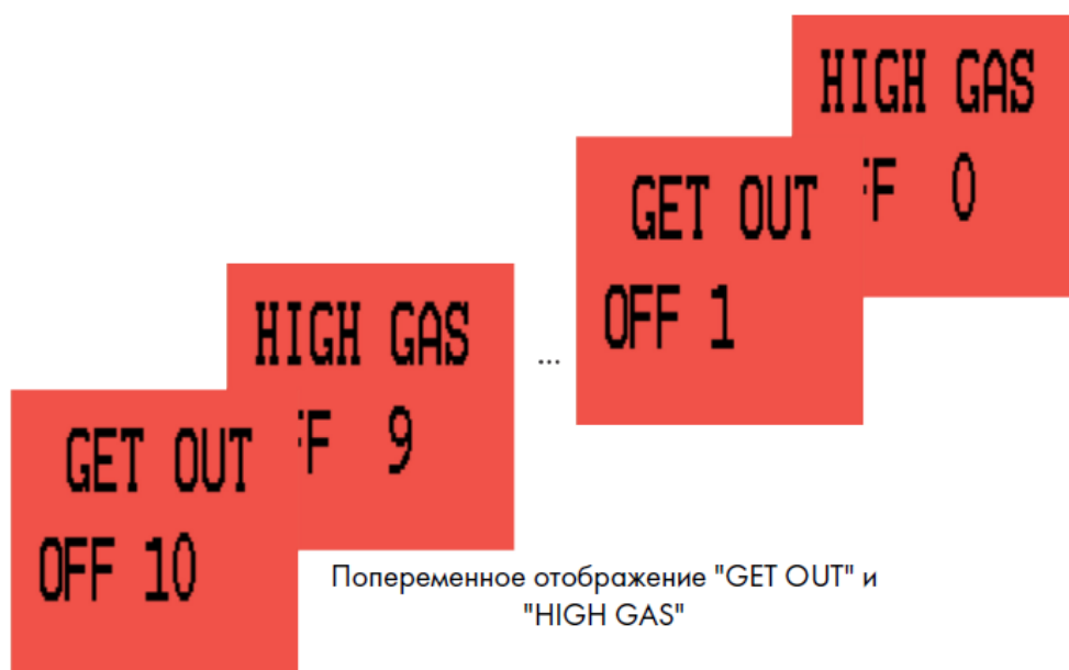
Рисунок 4-4: Таймер выключения GET OUT/HIGH GAS
