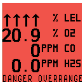
Рисунок 4-3: Сигнализация по выходу за пределы диапазона
