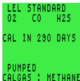
Рисунок 3-2: Режим быстрого просмотра настроек
