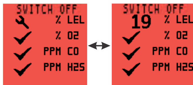
Рисунок 5-5: ZERO FAULT – SWITCH OFF (выключите прибор)
