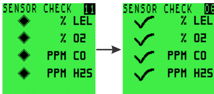
Рисунок 3-12: Экраны проверки датчиков
