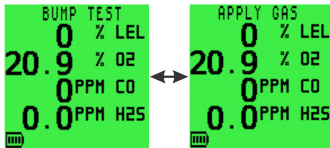
Рисунок 6-2: Экран подачи газа (4-канальная модель)
