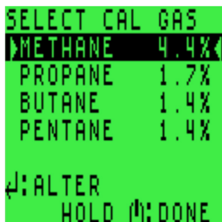
Рисунок 3-11: Выбор калибровочного газа
