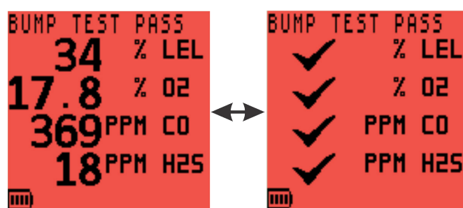
Рисунок 6-6: Контрольный замер пройден
