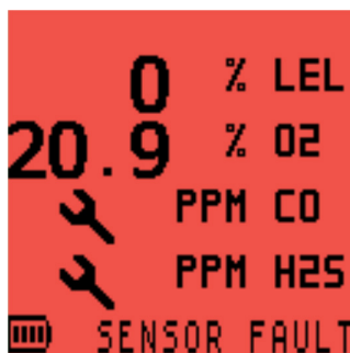
Рисунок 5-7: Отказ датчика CO/H 2 S
