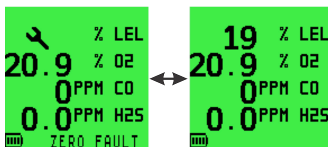
Рисунок 5-4: Сбой LEL ZERO
