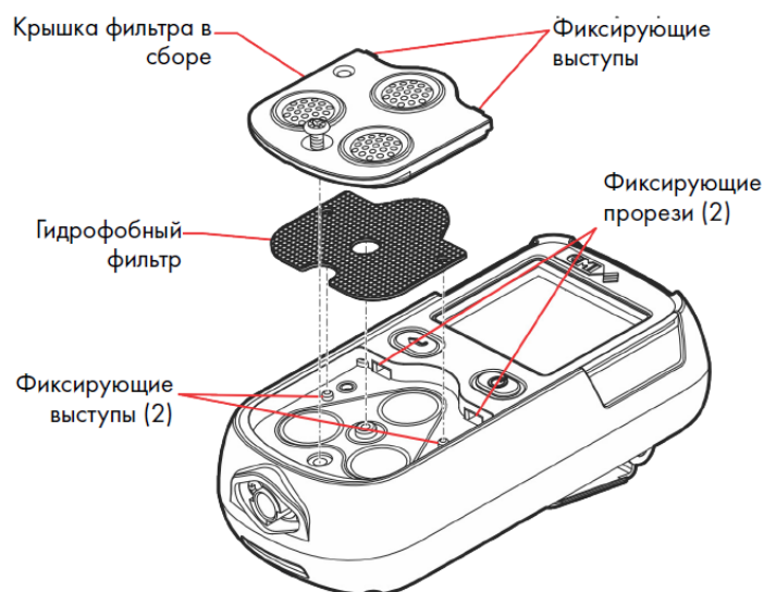
Рисунок 8-1: Замена гидрофобного фильтра
