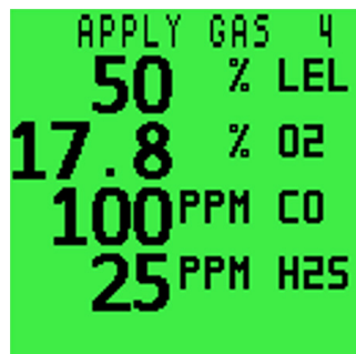
Рисунок 9-5: Экран APPLY GAS (подача газа)
