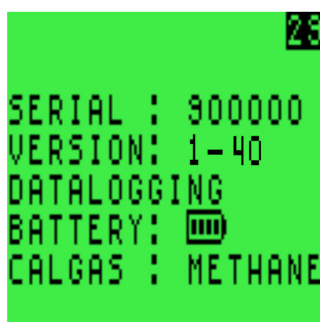
Рисунок 3-4: Экран идентификации газоанализатора
