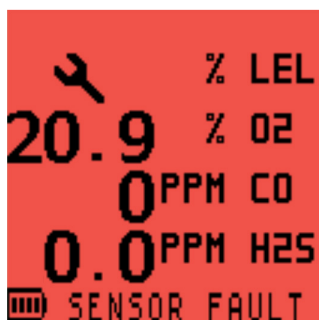
Рисунок 5-6: Отказ датчика НПВ
