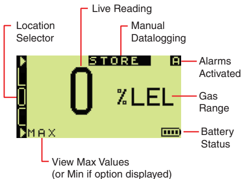
Fig. 1-2 CSM Button Press Options
