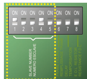
Figura 5 : interruptores de configuración de direcciones.
