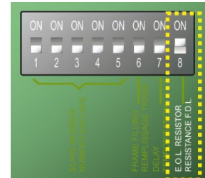
Figure 6: interrupteur de résistance de fin de ligne en position « ON »
