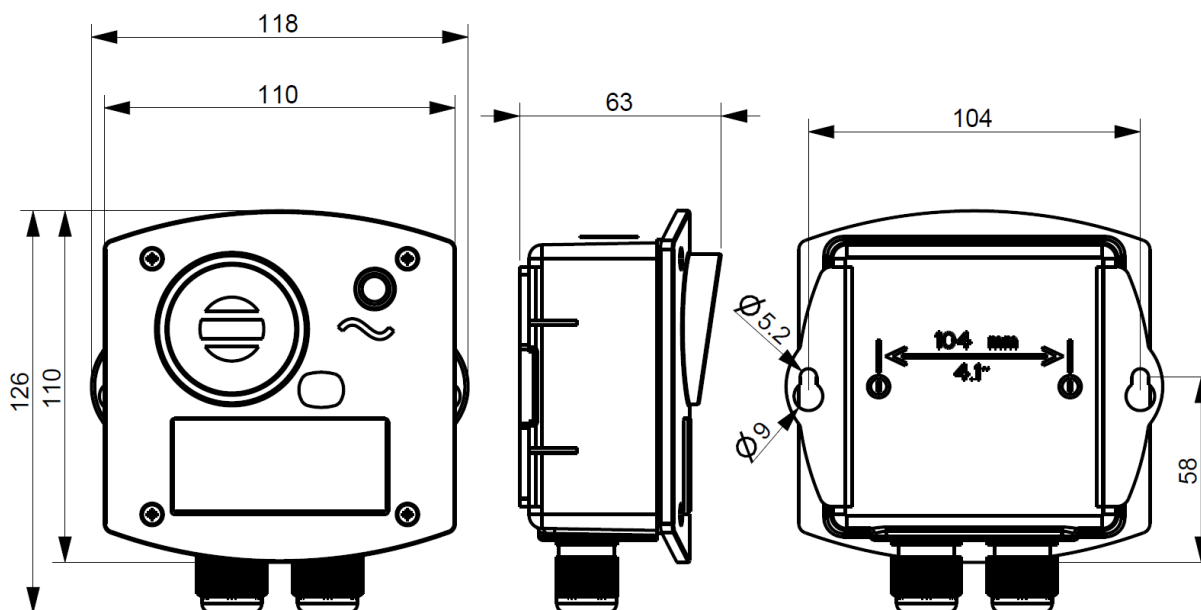
Figure 3: Encombrement de l'OLCT 10N (en mm)
