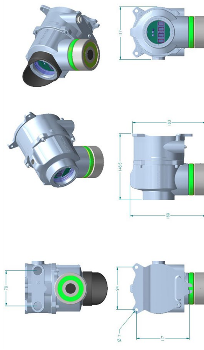
Figure 2 : Schémas d'encombrement (mm)
