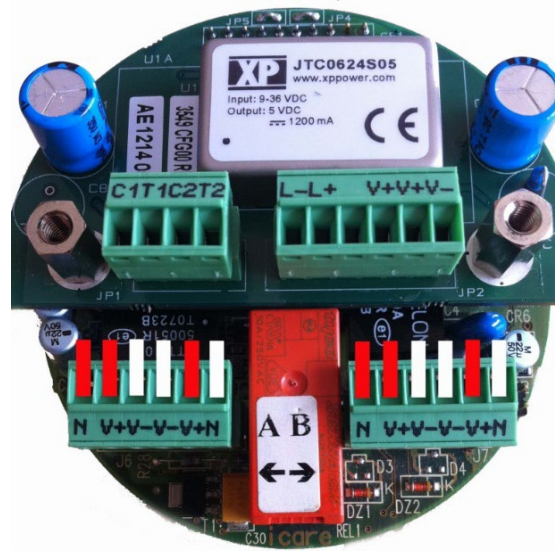
Figure 4 : Schéma de raccordement des versions réseau
