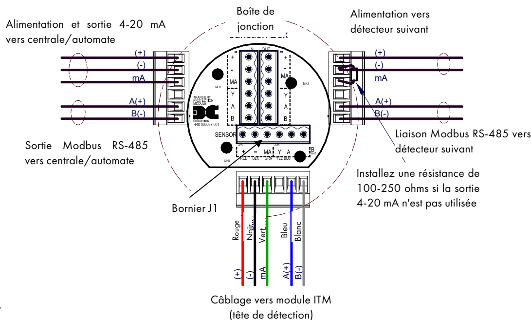
Figure 11 : Connexions
