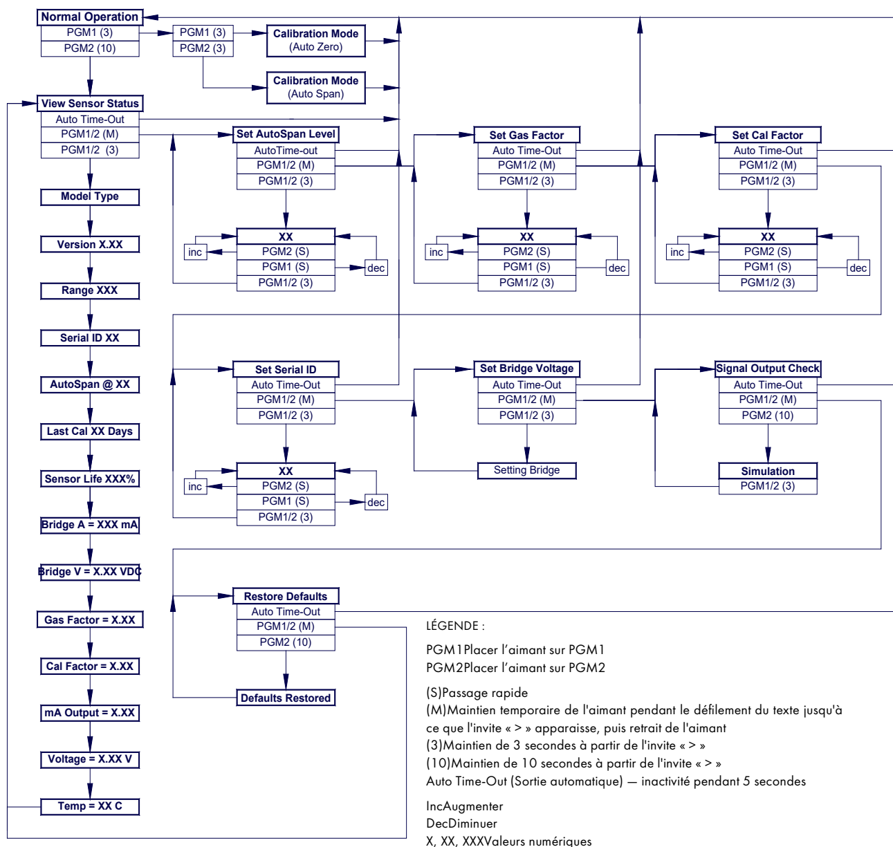
Figure 14 : Arborecence des menus OLCT 700/710 FP
