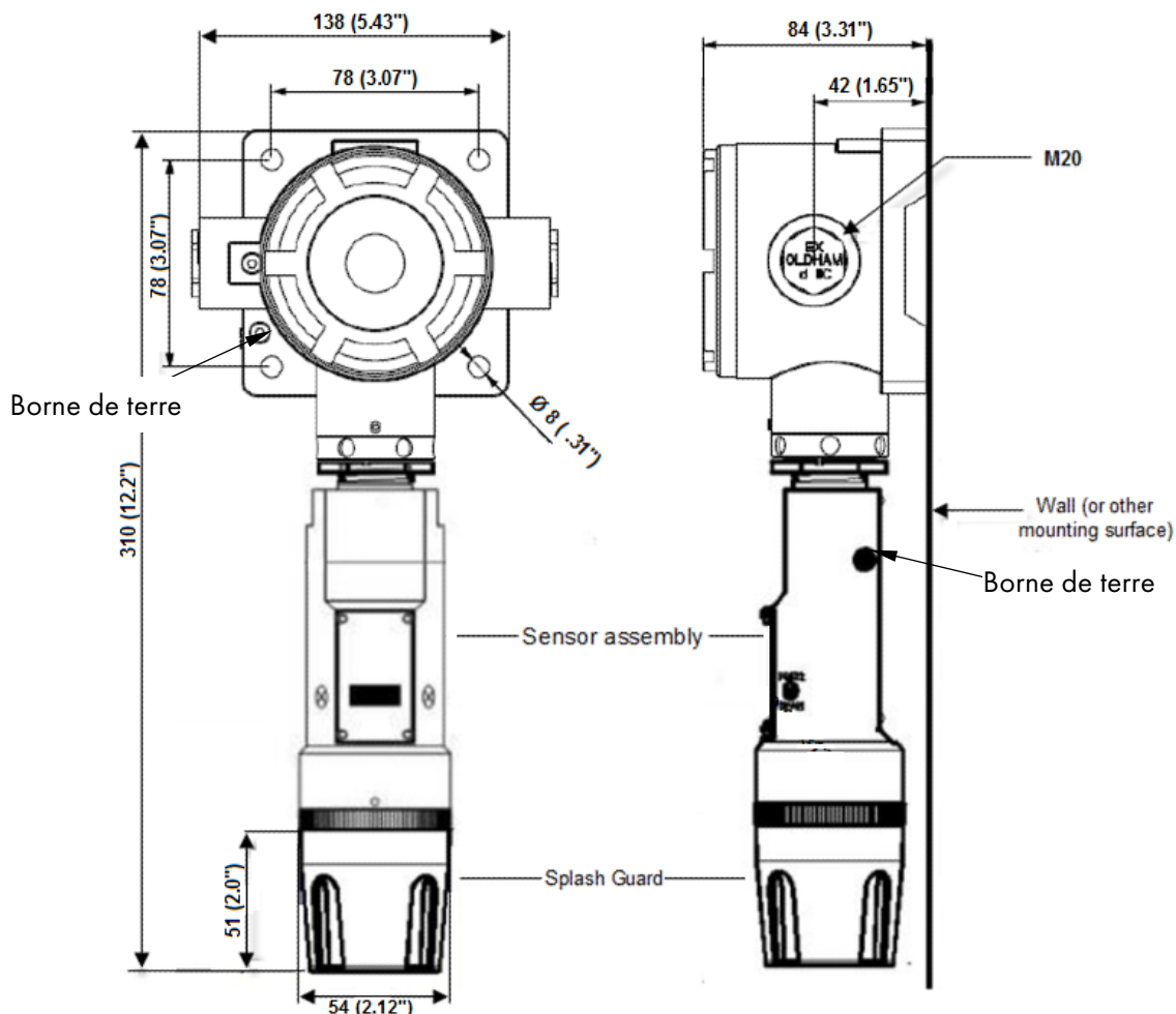
Figure 9 : Dimensions extérieures
