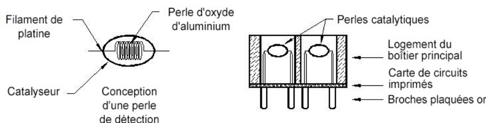
Figure 1 : Détecteur à perles catalytiques
