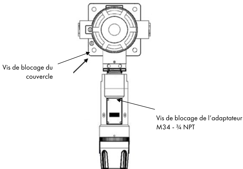
Figure 6 : Vue de face de l'OLCT 710
