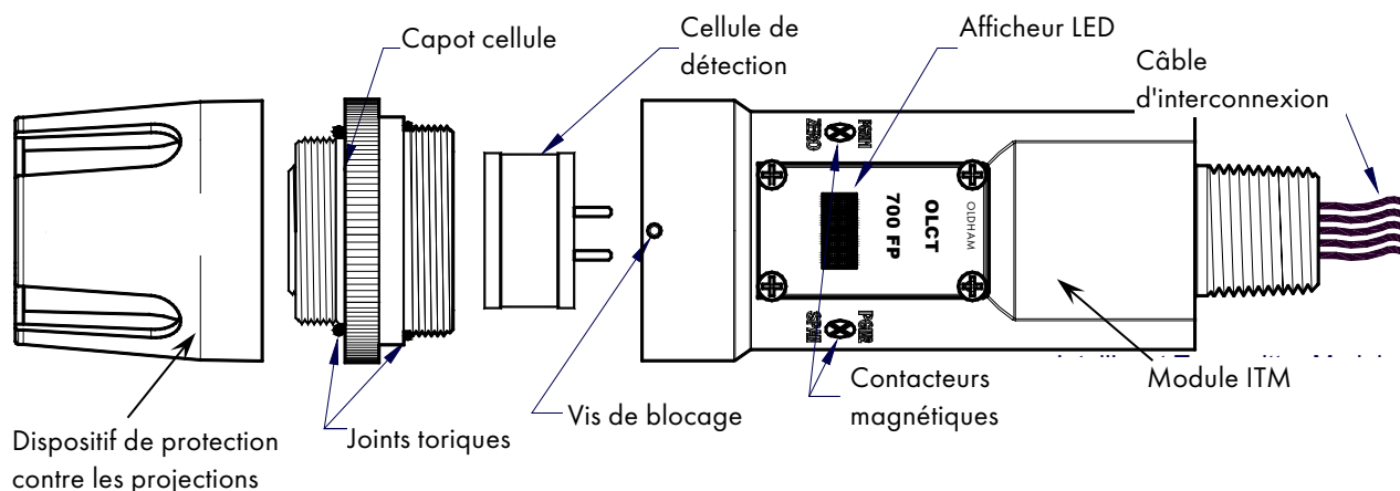
Figure 4 : Décomposition du détecteur
