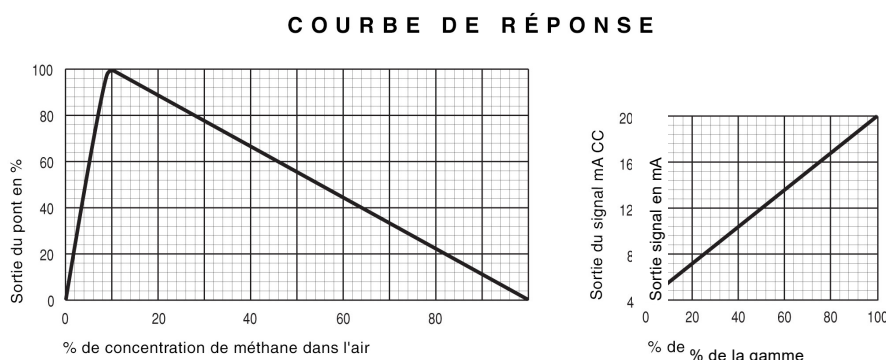
Figure 3 : Courbes de réponse
