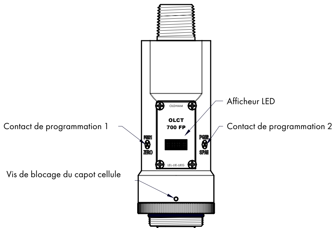
Figure 5 : Vue de face de l'OLCT 700
