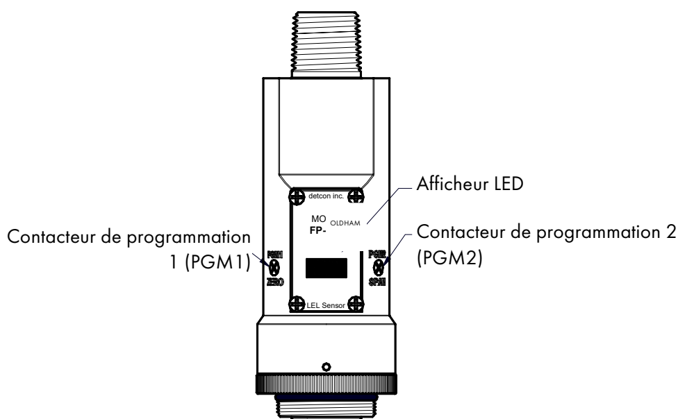
Figure 13 : Contacteurs magnétiques de programmation
