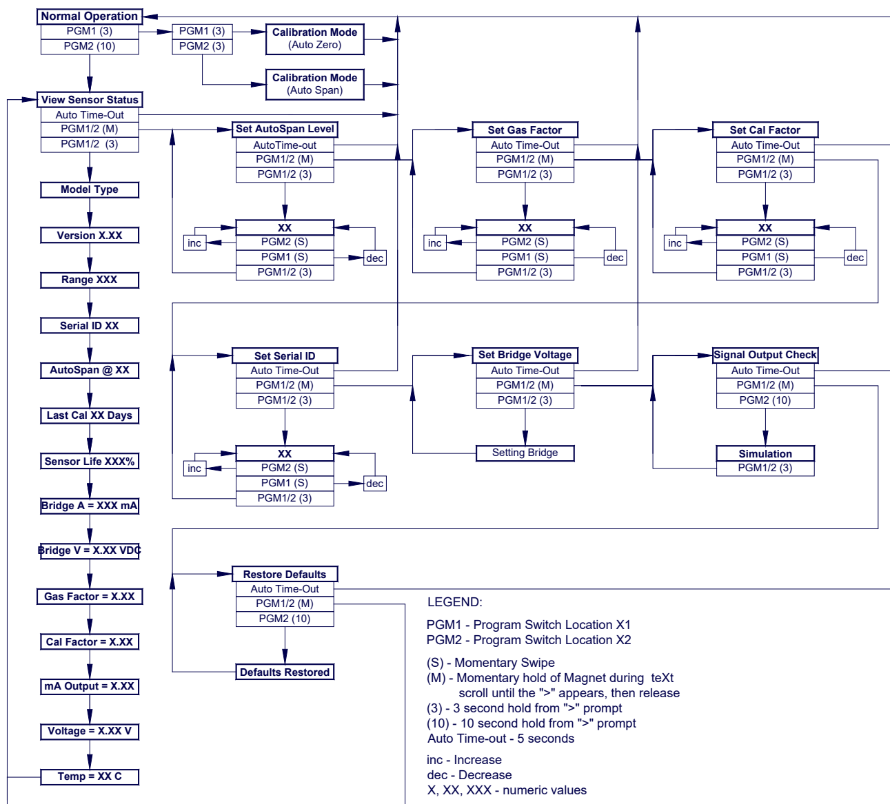
图 14: OLCT 700/710 FP 软件流程图
