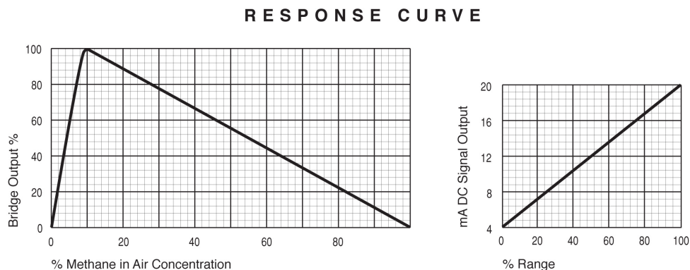
图 3: 响应曲线
