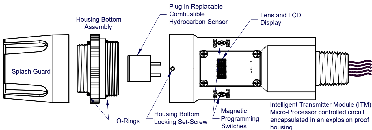
图 4: 检测仪组装分解图
