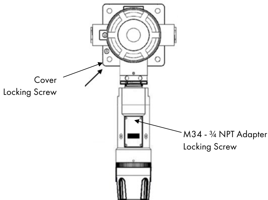
图 6: OLCT 710 前视图
