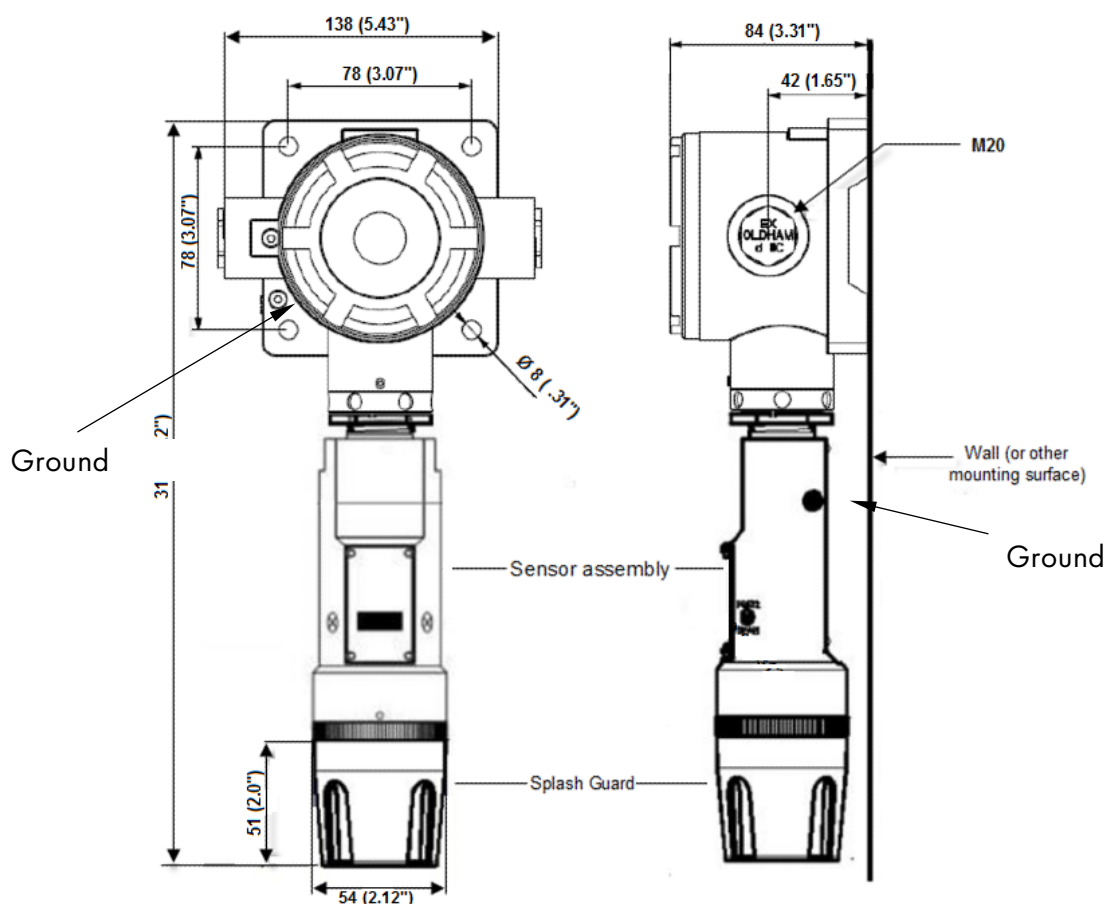
图 9: 外形和安装尺寸
