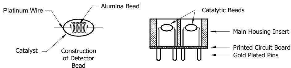
图 1: 传感器内部结构
