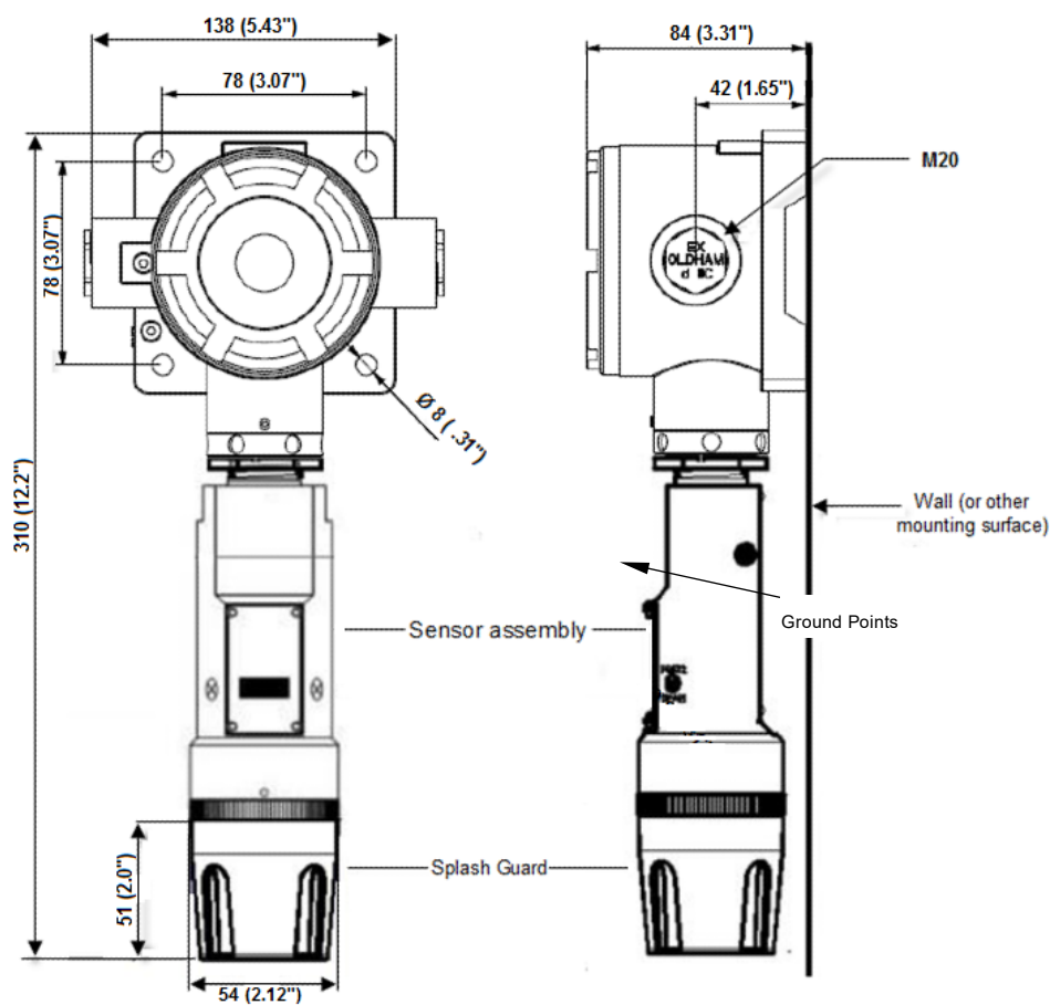
OLCT 710 FP 尺寸图
