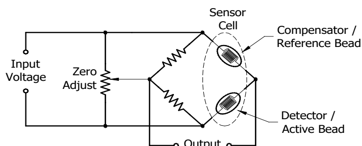
图 2: 惠斯通电桥
