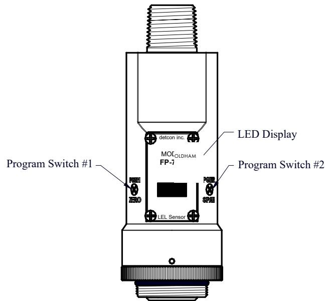
图 13: 磁性编程开关
