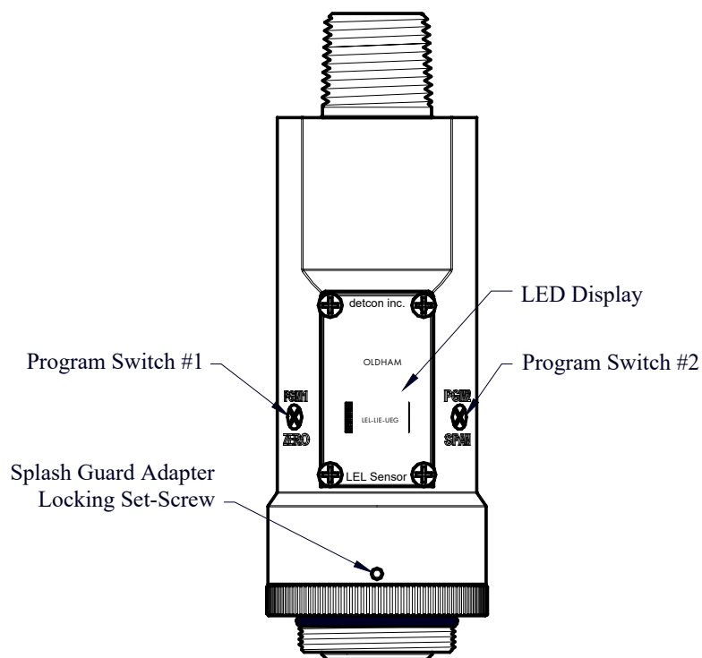
图 5: OLCT 700 组件前视图
