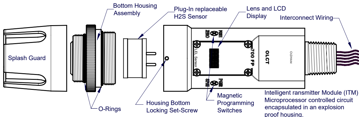
图 15: 传感器组装图
